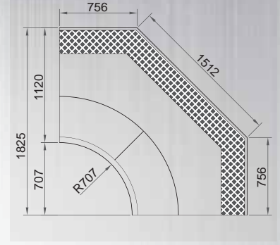
GARDENYA 112 - 90° İç Köşe GARDENIA 112 - 90° Internal Corner
