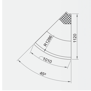
GARDENYA 112 - 45° Dış Köşe GARDENIA 112 - 45° External Corner
