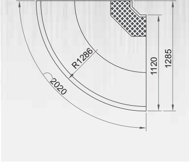
GARDENYA 112 - 90° Dış Köşe GARDENIA 112 - 90° External Corner
