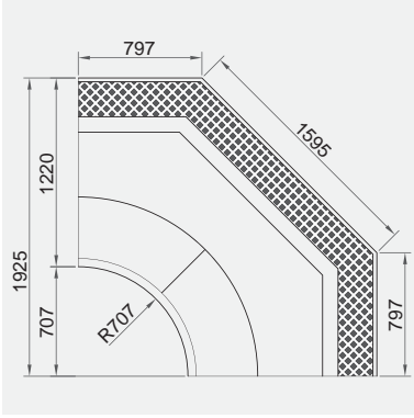
GARDENYA 122 - 90° İç Köşe GARDENIA 122 - 90° Internal Corner
