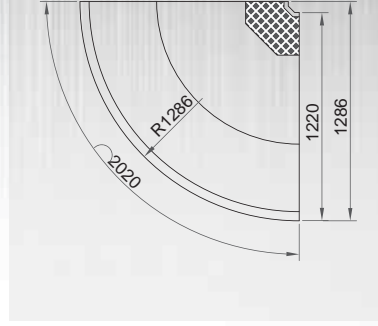
GARDENYA 122 - 90° Dış Köşe GARDENIA 122 - 90° External Corner
